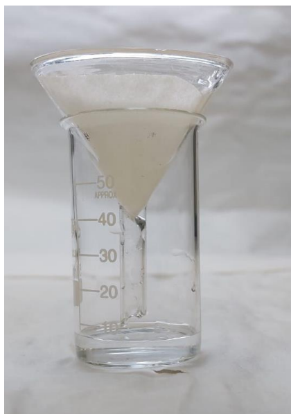
Рисунок 8 – Фильтрация горячего насыщенного раствора борной кислоты
