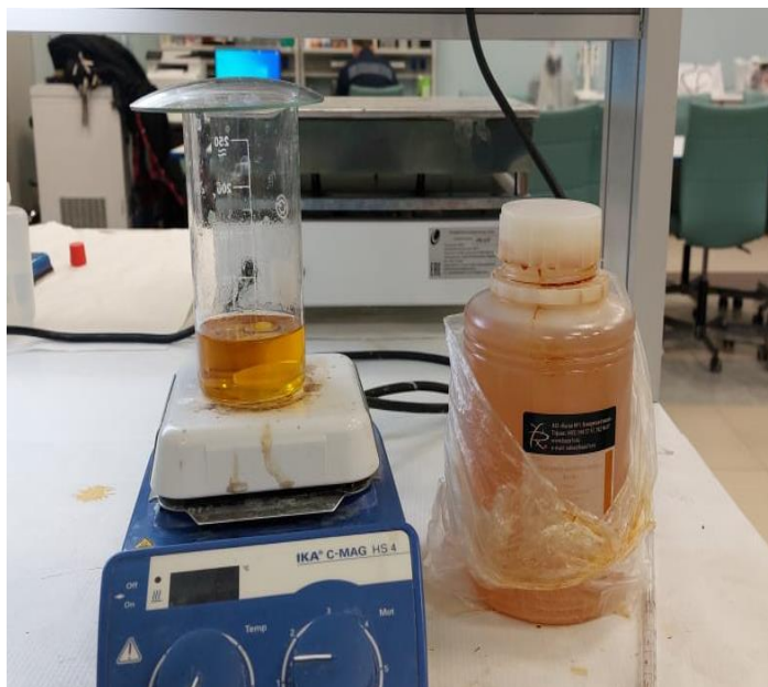
Рисунок 17 – Получение связующего компонента пасты для вжигания
