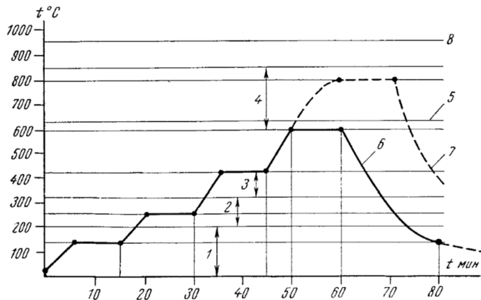
Рисунок 2 – График зависимости времени протекания процесса вжигания от температуры обжига.
